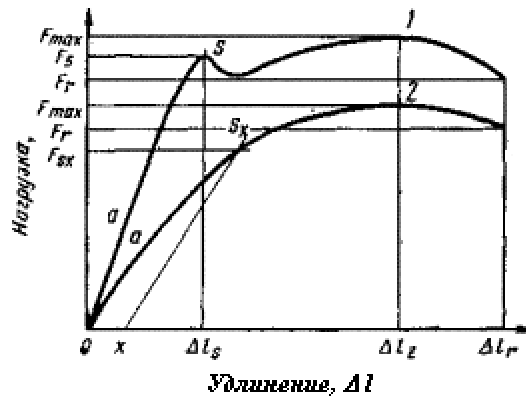
1—материал имеет предел текучести; 2—материал не имеет предела текучести; а—участки прямолинейного направления кривой в начале кривой «нагрузка-удлинение»; S—предел текучести; x—отрезок на оси удлинения для определения условного предела текучести; S x —условный предел текучести Черт. 5
